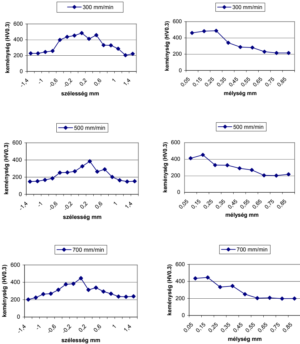
3.23. ábra Keménységeloszlás az átolvasztott sáv szélességében, mélységében különböző pásztázósebesség mellett (a lézerrugár teljesítménye 1 kW)
