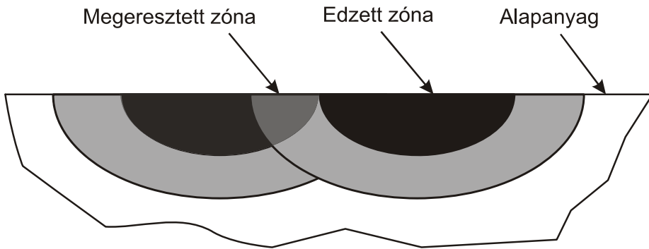
2.25. ábra Átlapolódó nyomvonalak egymásra hatása
