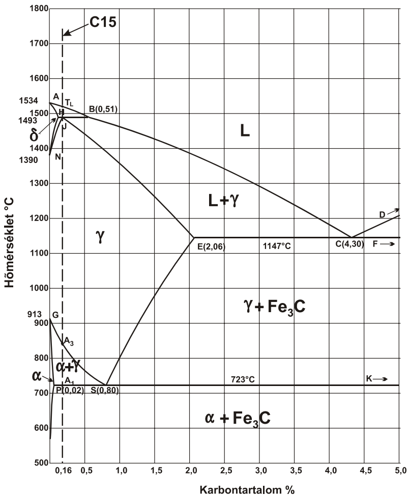
3.2. ábra Fe-Fe 3 C diagram a vizsgált acél (0,16% C) összetételével
